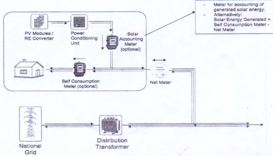
চিত্র ১: একটি আদর্শ নেট মিটারিং সিস্টেম
