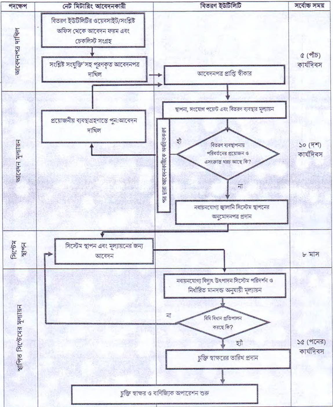
চিত্র ২: নেট এনার্জি মিটারিং আবেদনপত্র প্রক্রিয়াকরন
