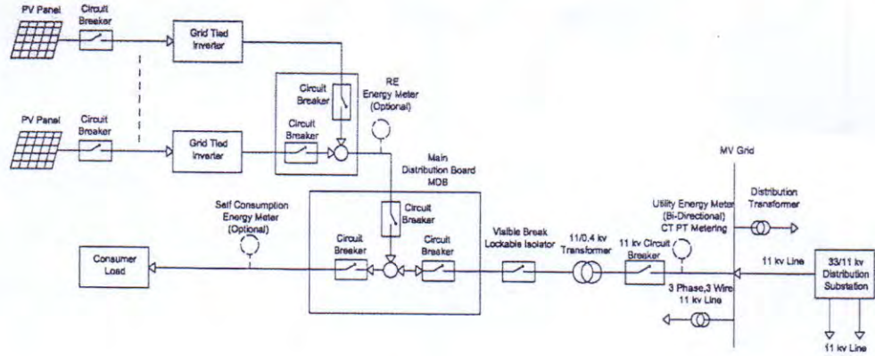
চিত্র ৫: টাইপ B সংযোগ (MV গ্রাহক)
