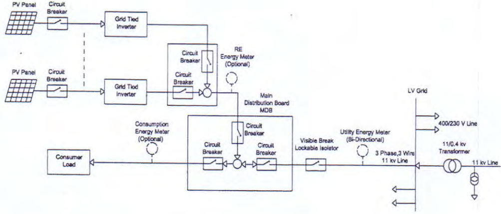
চিত্র ৪: টাইপ A বৈদ্যুতিক সংযোগ (LV গ্রাহক)
